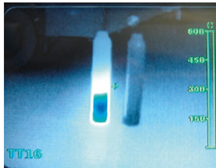
Füllstand Gasflasche
